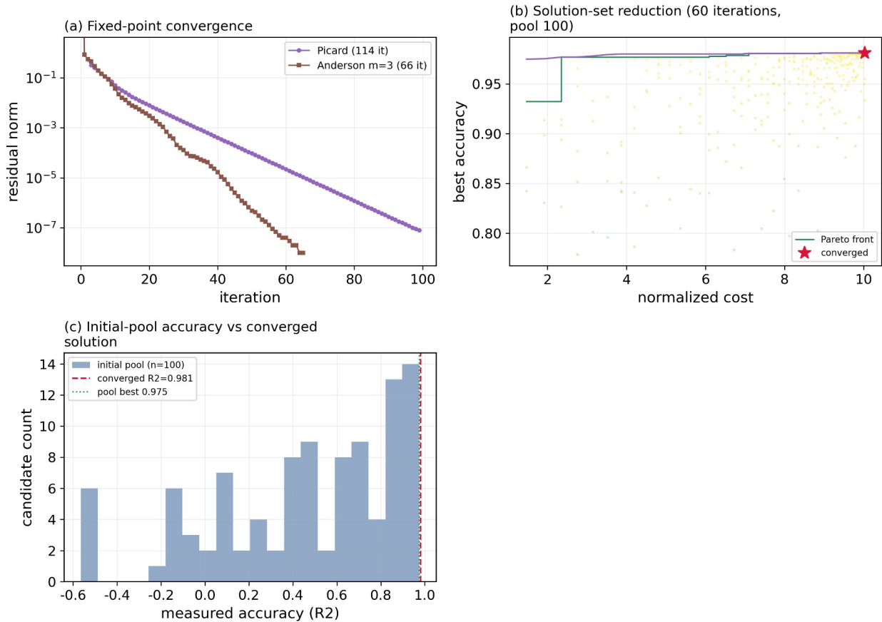
그림 5. 해공간 탐색과 수렴 거동. (a) Anderson 가속과 Picard 반복의 잔차 수렴 비교; (b) 해집합 축소 반복의 후보윤·비지배 전선과 최고 정확도 수렴 궤적; (c) 초기 후보 풀(전수 실행) 정확도 분포와 수렴 차기 해의 개선도.
