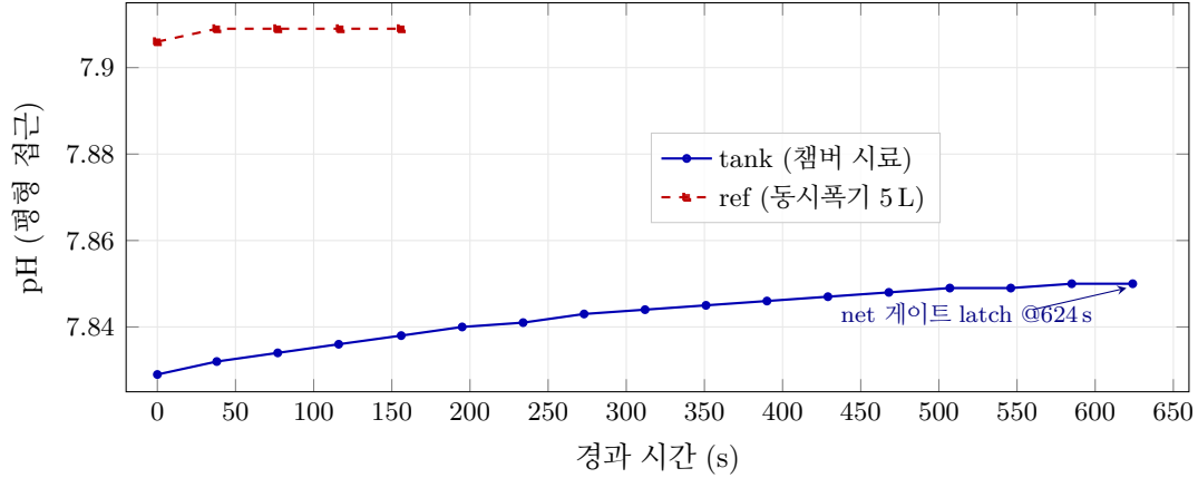
Figure 2: 실측 평탄 추종 곡선(밀폐, net 게이트 실행). tank 시료(실선)는 느린 지수 꼬리를 등반하며 이중 게이트 판정(최근 4개 \text{span} \leq 2\text{mPH} 및 최근 8개 \text{net} \leq 1\text{mPH} )이 충족될 때만 latch된다; 동시폭기된 참조수(점선)는 이미 평형 근처라 빠르게 latch된다. 두 계열의 pH가 다른 것은 기저 시료가 다르기 때문이며(이 실험은 널 캠페인 이전), 각자의 평탄 값만이 식 (3)에 들어간다.
