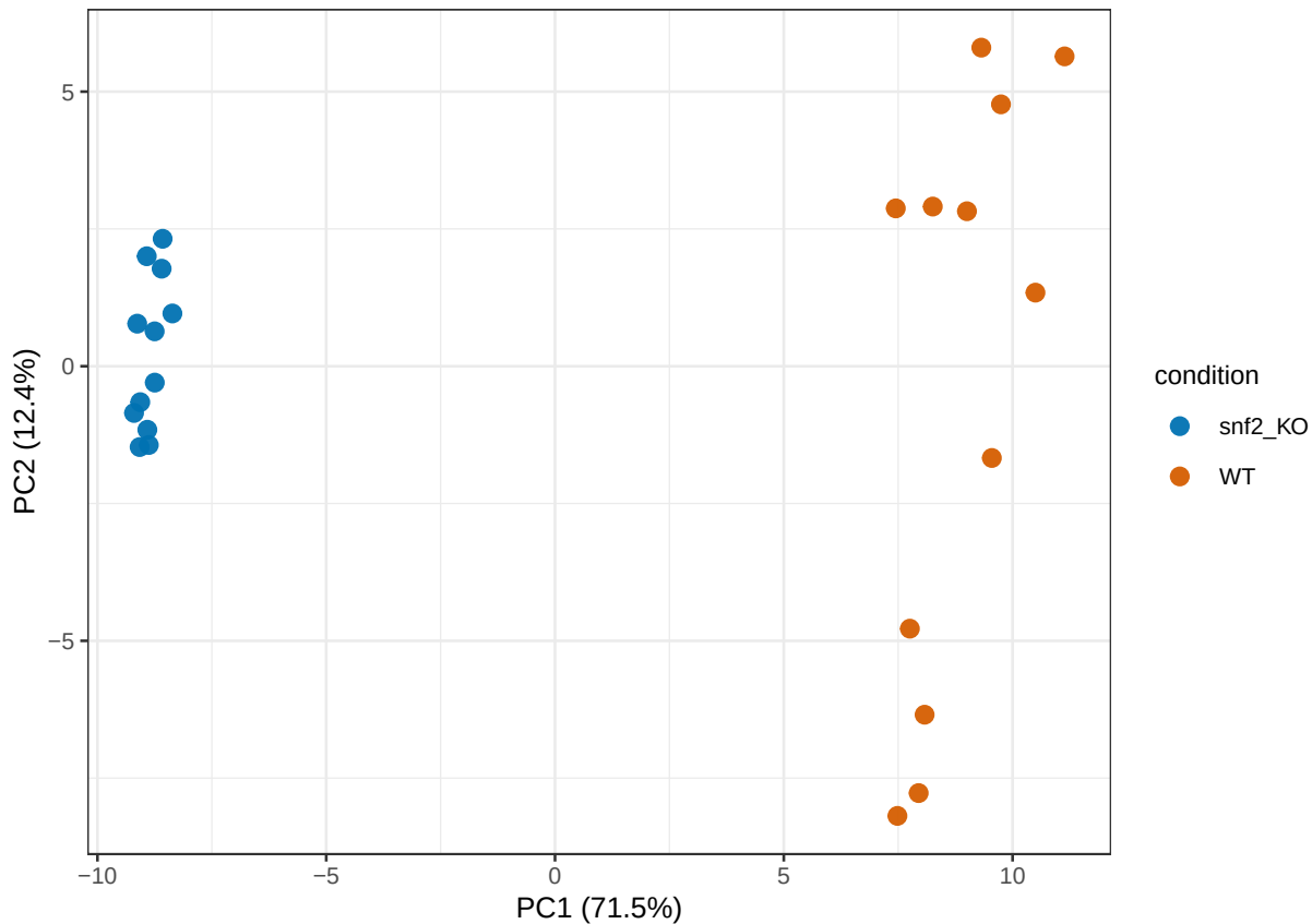
PCA of VST expression
