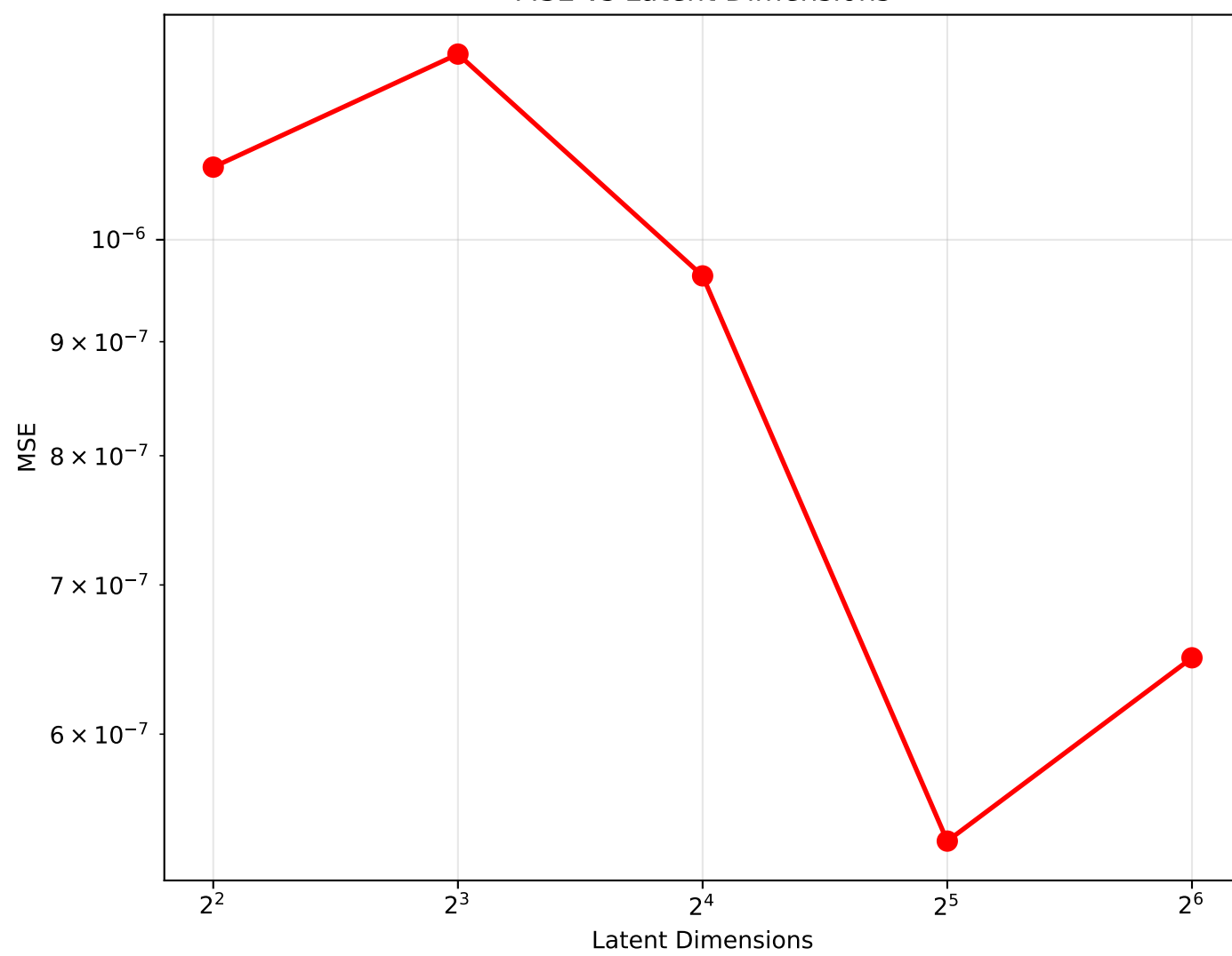
MSE vs Latent Dimensions
