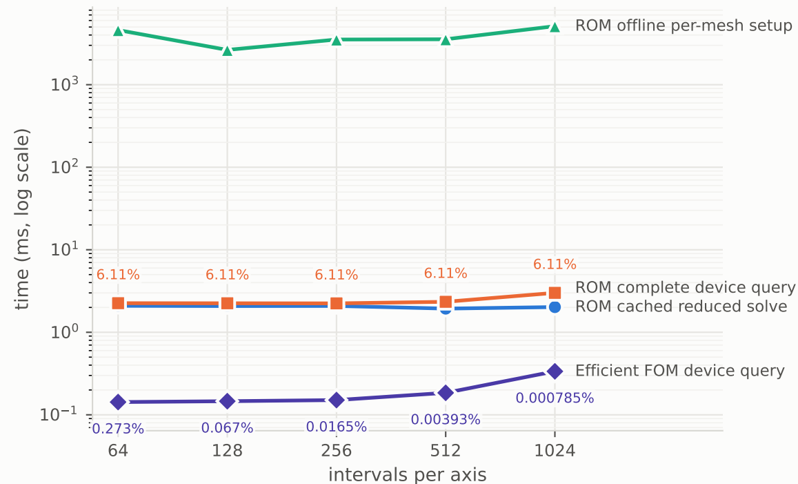
Poisson 2D
