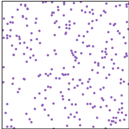
Monte Carlo m = 256
