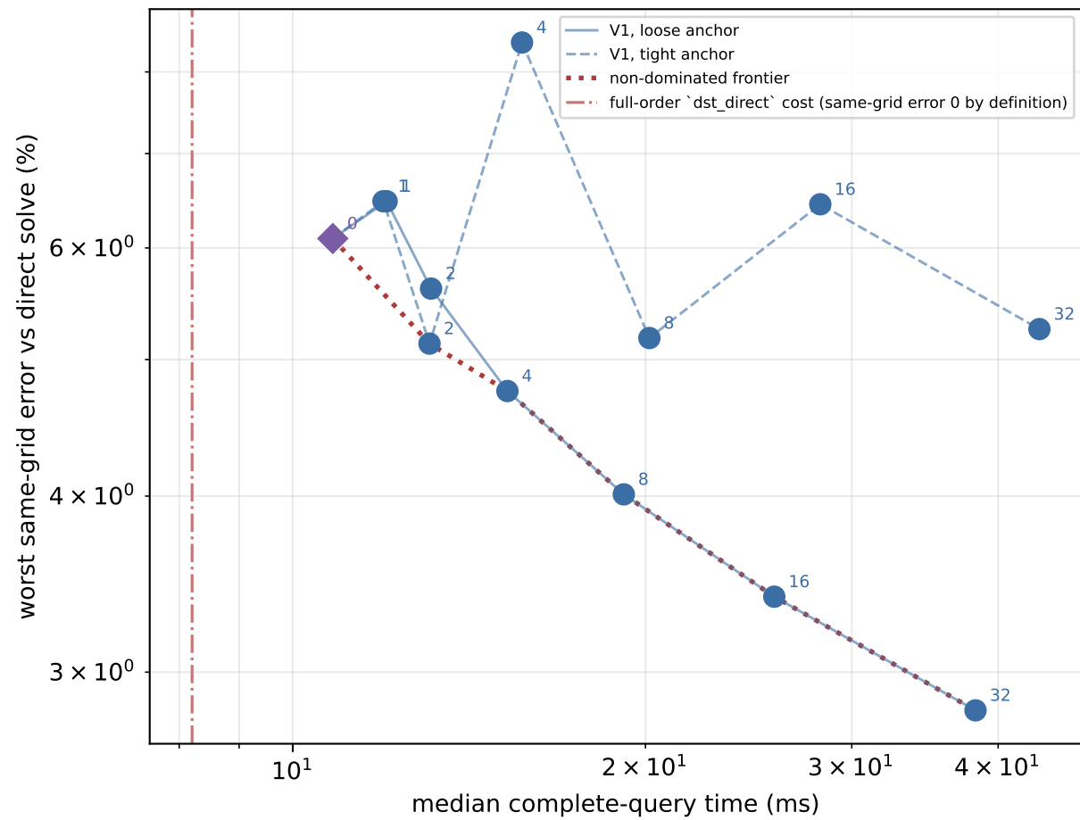
Poisson 2D, 1024 intervals (V1 only; V2 collapses onto it)
