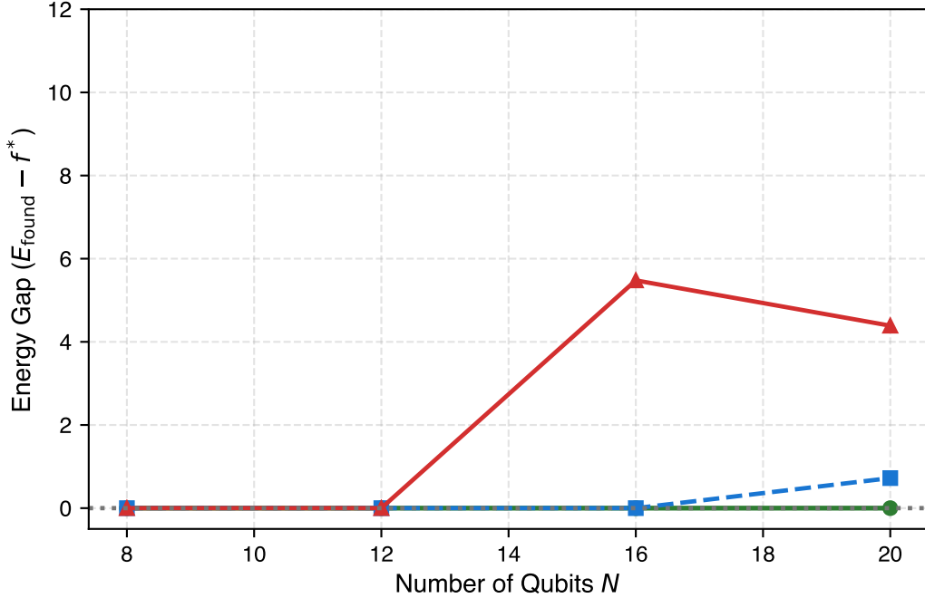
(d) Optimality Gap to Ground Truth vs Scale N
