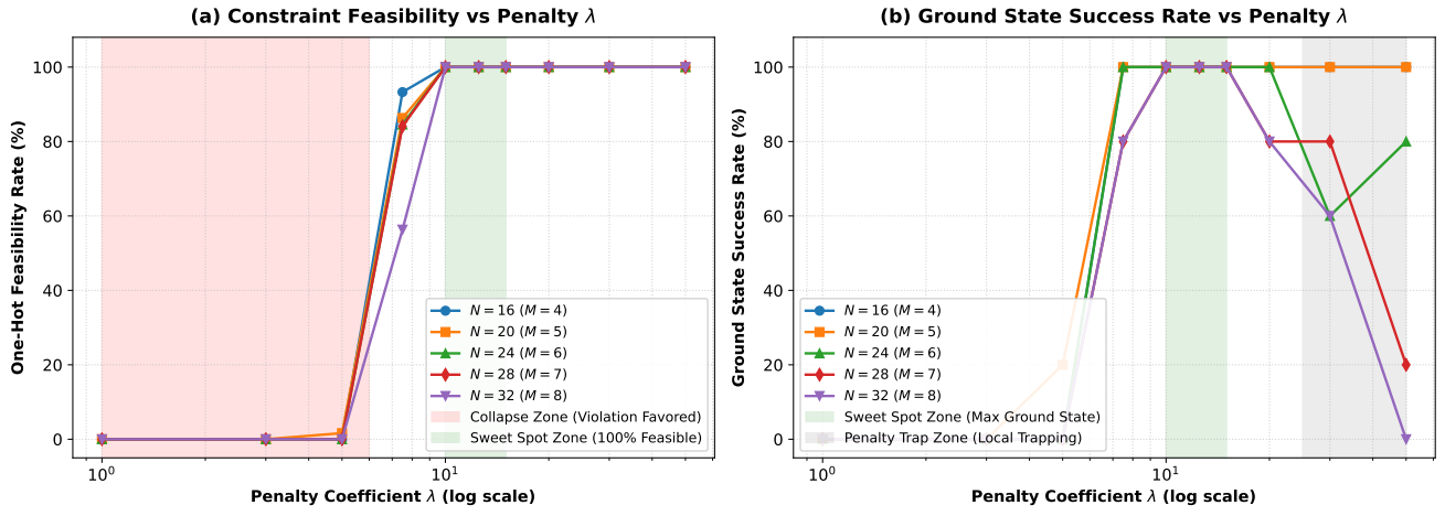
図 2: FMQA におけるペナルティ係数 \lambda のスイートスポット解析：(a) 制約充足率の立ち上がり（崩壊ゾーン vs 充足ゾーン），(b) 真の大域最適解到達率の山型変化（スイートスポット [10, 15] と過大ペナルティによる探索性能劣化）。
