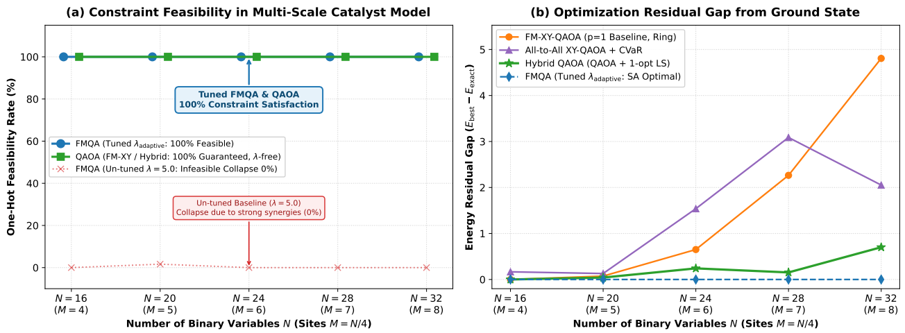
図 1: 多元触媒モデルにおけるスケーリング特性の比較 (更新版): (a) One-Hot 制約充足率 (固定ペナルティ \lambda = 5.0 の破綻 vs 適応型 FMQA および QAOA の 100% 完全防衛), (b) 真の大域最適解に対するエネルギー残差ギャップの推移 (Hybrid QAOA による劇的な高精度化と SA への肉薄).
