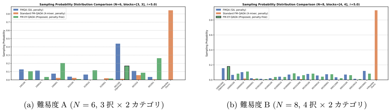
図 2: サンプリング確率分布の比較 ( \lambda = 5.0 )。Standard QAOA (橙) は右端の無効解に大半の確率が流出している。提案手法 (緑) は無効解がゼロであり、最適解 x^* (黒棒) に高い確率が集中している。
