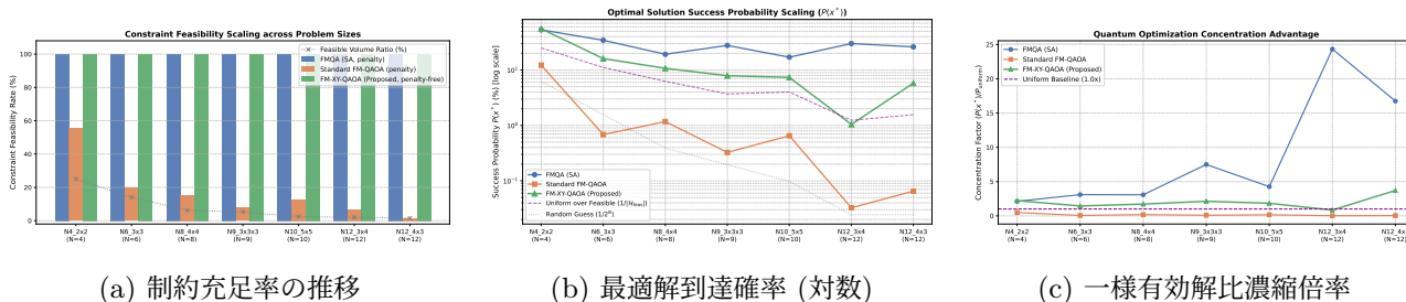
図 1: 7 段階の問題スケールにおける性能スケーリングの比較。(a) Standard QAOA は指数関数的に崩壊するのに対し提案手法は 100% を維持。(b) 提案手法は一貫して Standard QAOA を圧倒。(c) 一様サンプリングに対する濃縮効果を実証。
