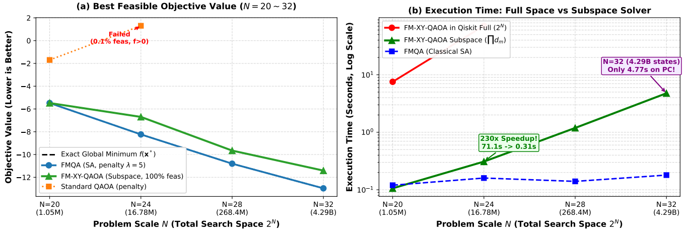
図 2: 大規模直接対決実測結果 ( N = 20 \sim 32 )。 (a) 最良目的関数値推移。Standard QAOA は N \geq 24 で正の値に脱線し完全破綻するが、FM-XY-QAOA は厳密最適解の近傍を確実に捕捉。 (b) シミュレーション実行時間。Qiskit 全空間では N = 24 で 71 秒を要したが、部分空間ソルバーにより N = 24 で 0.31 秒 (230 倍高速化)、 N = 32 (42.9 億次元) でもわずか 4.77 秒で完了した。
