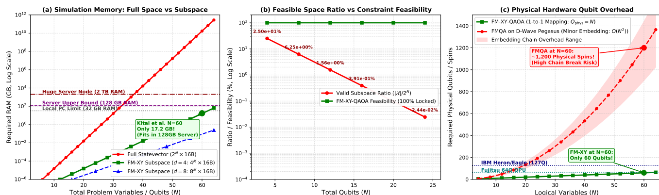
図 1: 対称性によるスケーリング限界突破とハードウェア・変数比較の徹底対比。(a) シミュレーション所要メモリ推移。全空間 (赤) は N \geq 32 でサーバー限界を突破し N = 60 で 18.4 EB に達するが、部分空間 (緑) は N = 60 でも 17.2 GB に抑えられ 128GB サーバーで実行可能。(b) 有効解比率と制約充足率。Standard QAOA は 0% へ死滅するが、提案手法は全域で 100.0% を完全堅持。(c) ハードウェア物理量子ビット数。FMQA (アニーリング) は Minor Embedding により O(N^2) で激増するが、提案手法は 1 対 1 ( Q_{phys} = N ) で極めて省リソース。
