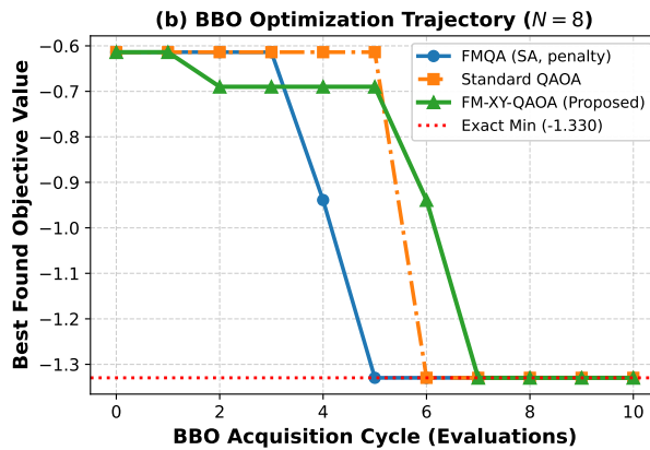
図 1: N = 8 相互作用 BBO 探索推移。提案手法 (緑) は制約違反ゼロで大域最適解 ( -1.330 ) へ収束。
