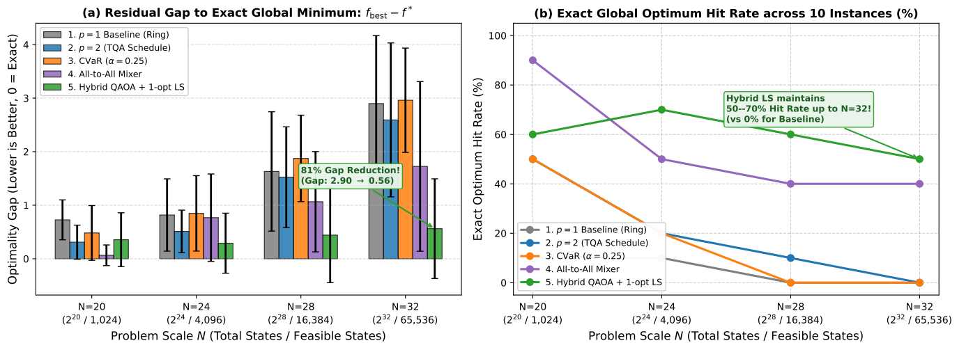
図 3: QAOA 精度向上策の実測比較結果 ( N = 20 \sim 32 、各 10 インスタンス)。(a) 厳密最適解との残差ギャップ推移。Hybrid 局所探索により N = 32 (42.9 億通り) でもギャップが 2.90 \rightarrow 0.56 へと 81% 激減。(b) 厳密大域最適解到達率 (Hit Rate)。Baseline が規模拡大で 0% に低下する中、全結合ミキサーや Hybrid 手法は極大スケールでも 40–50% の高い成功率を堅持した。
