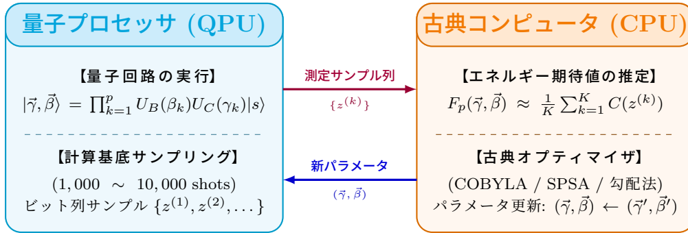
図 4.2 QAOA における量子・古典ハイブリッド最適化ループ (VQE/VQA 型). QPU が量子重ね合わせから高速にサンプルを生成し, 古典 CPU がエネルギーを評価してパラメータ (\vec{\gamma}, \vec{\beta}) を更新する.
