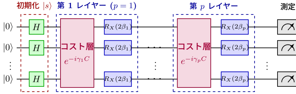
図 4.1 QAOA の全体量子回路構成図. 全ビットへのアダマールゲート H で一様重ね合わせを作った後, コスト層 e^{-i\gamma C} とミキサー層 e^{-i\beta B} を p 回交互に適用し, 最後に計算基底で測定してビット列サンプルを得る.
