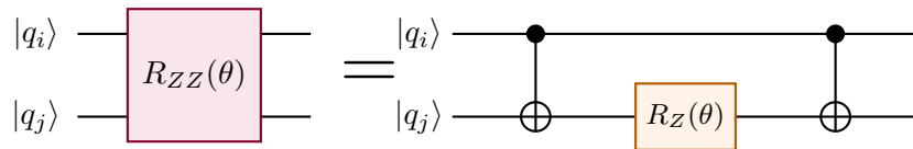
図 2.3 2 量子ビットイジング相互作用ゲート R_{ZZ}(\theta) = \exp\left(-i\frac{\theta}{2}Z_iZ_j\right) の標準的ゲート分解. 最初の CNOT でパリティ (2 ビットの排他的論理和) を標的に集約し, R_Z で位相を回転させた後, 2 つ目の CNOT で標的の状態を元に戻す.
