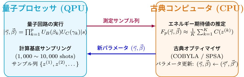
図 4.2 QAOA における量子・古典ハイブリッド最適化ループ (VQE/VQA 型). QPU が量子重ね合わせから高速にサンプルを生成し, 古典 CPU がエネルギーを評価してパラメータ (\vec{\gamma}, \vec{\beta}) を更新する.
