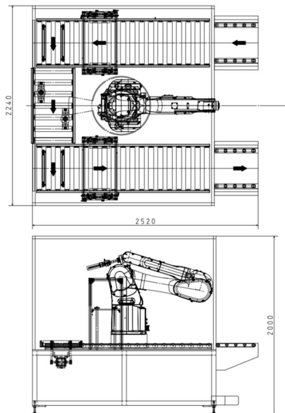
納入時寸法
