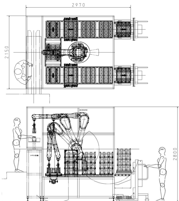
設備単体図
