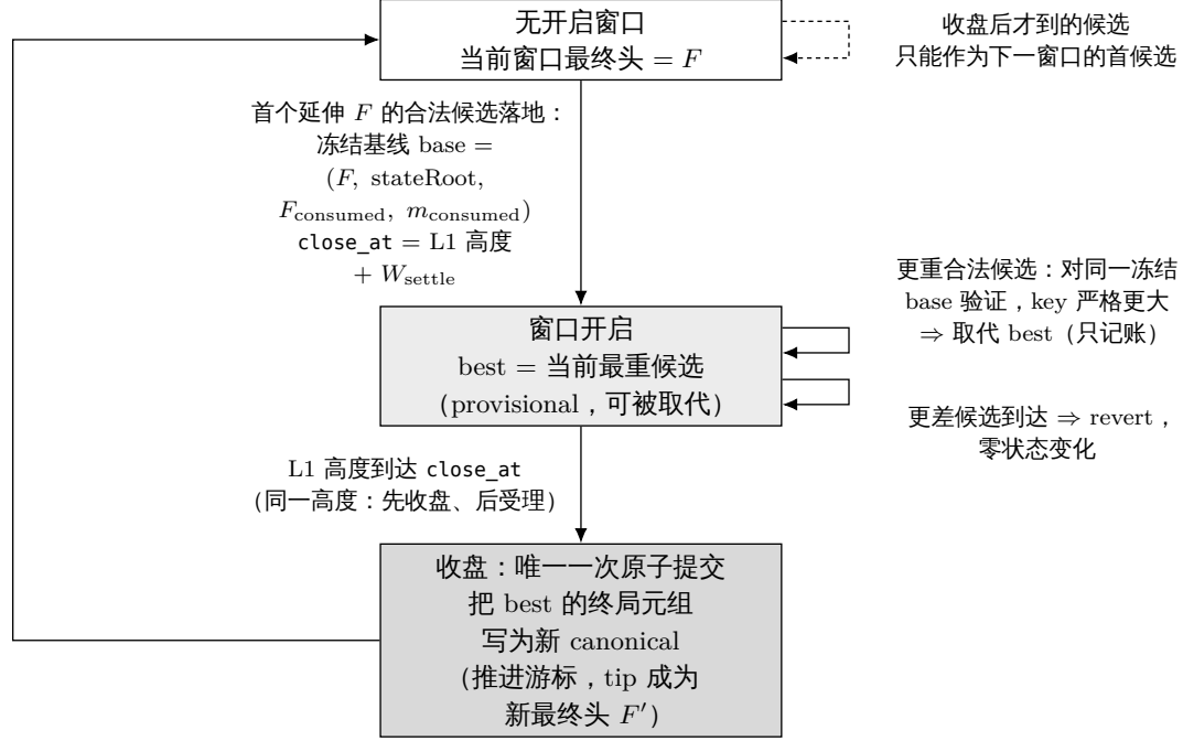
图 5: 结算窗口的生命周期状态机：窗口开启即冻结基线，窗口内所有候选对同一基线验证且只记账，直到收盘时才把最重候选的终局元组一次性原子提交为新的 canonical 状态。
