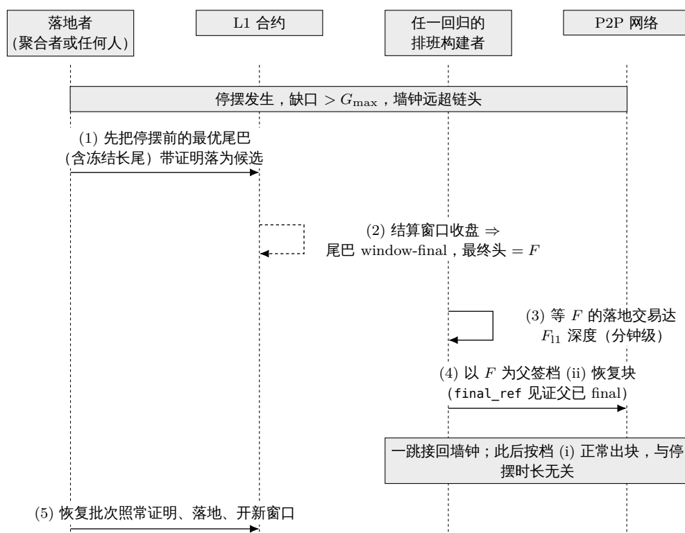
图 8: 数小时乃至数天停摆后的恢复时序：先把停摆前的最优尾巴落地并收盘为最终头 F ，再由任一回归构建者以 F 为父出一个档 (ii) 恢复块，一跳把排序接回墙钟，恢复过程不含独立子协议。
