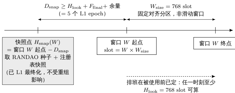
图 3: 快照点、排班窗口与前瞻视界的时间几何：熵与注册表在窗口起点前 D_{\text{snap}} 处一次性冻结，因而任一时刻均有至少一个完整窗口的排班可被任何人计算。
