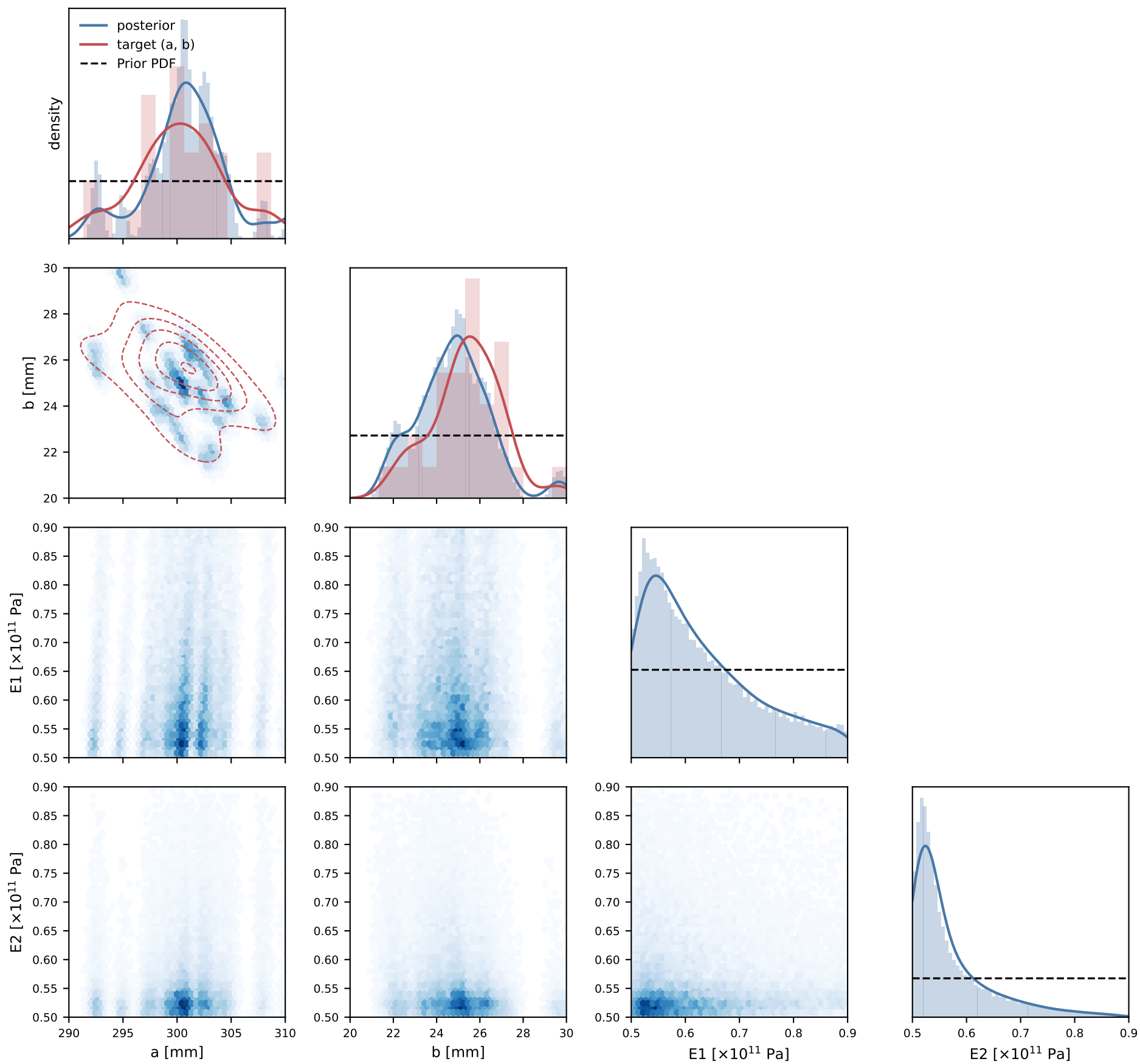
cDDPM | pooled posterior vs target (histogram + KDE)
