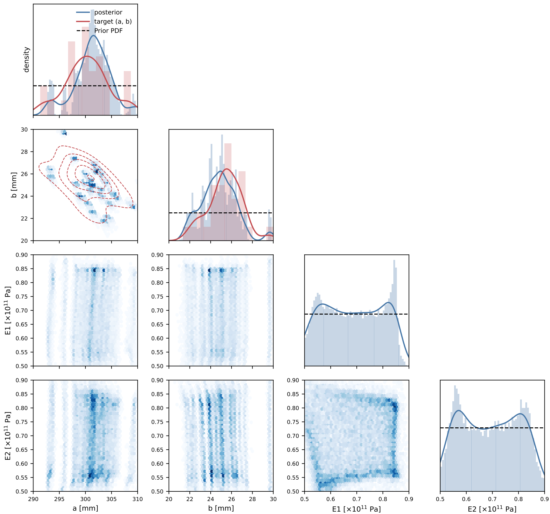
cGAN | pooled posterior vs target (histogram + KDE)
