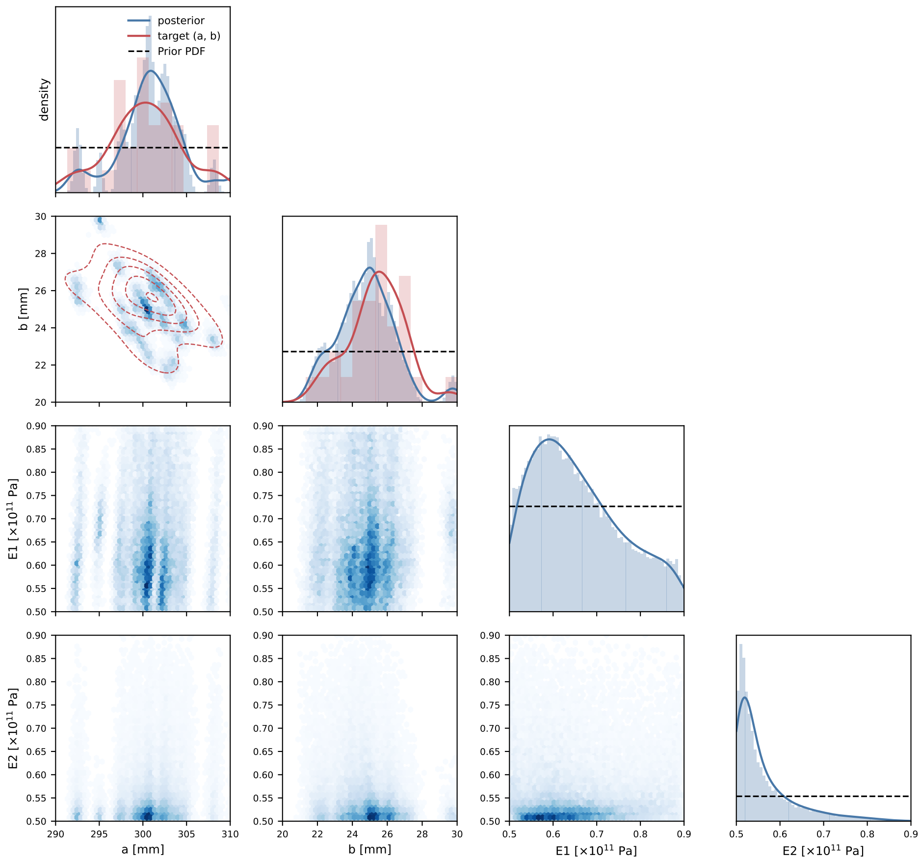
cNF | pooled posterior vs target (histogram + KDE)
