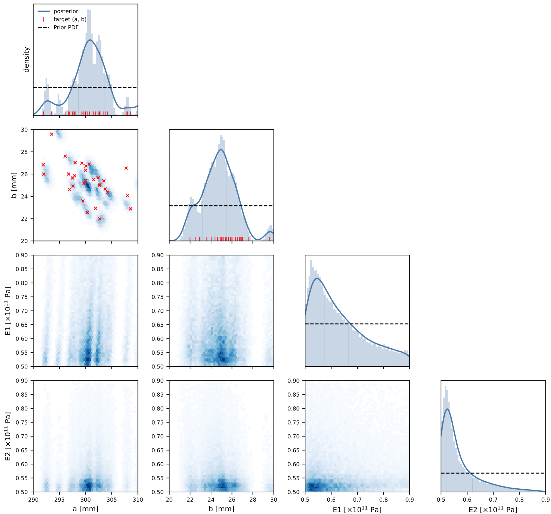
cDDPM | pooled posterior (histogram)
