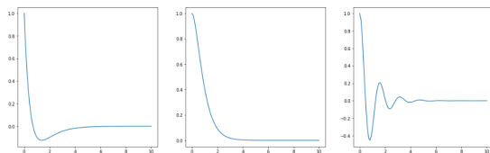
図 1.1: 例題 8 のグラフ
