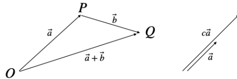
図 1.4: ベクトルの和（左）とスカラー倍（右）
