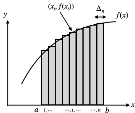
図 1.7: 1次元積分の概念図
