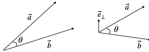
図 1.5: ベクトルの内積（左）とベクトルの外積（右）
