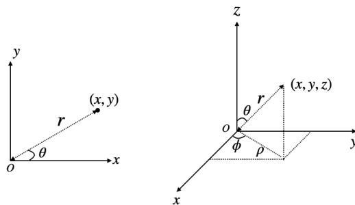
図 1.6: 2次元極座標（左）と3次元極座標と円筒座標（右）
