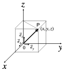
図 1.3: 3次元直交座標系でのベクトルと基底ベクトル
