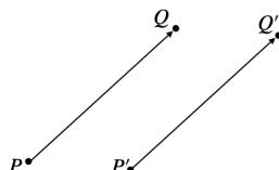
図 1.2: \vec{PQ} と \vec{P'Q'} は同じ向きで同じ長さの有向線分であるので、同じベクトルとみなされる。
