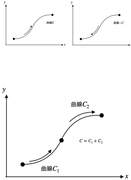
図 1.9: 線積分の性質
