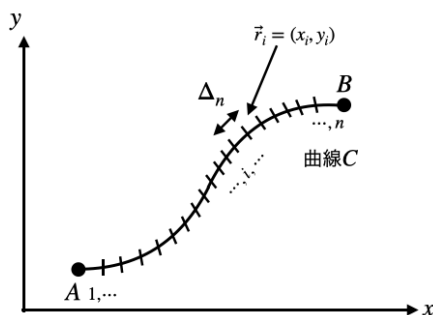
図 1.8: 線積分の概念図
