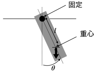
図 10.2: 物理振り子の模式図
