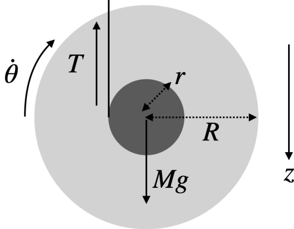
図 10.4: ヨーヨーの模式図
