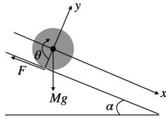
図 10.3: 斜面を転がる円筒の模式図
