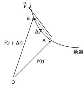
図 2.3: 質点の速度
