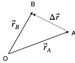
図 2.2: 質点の運動の変位と位置ベクトル
