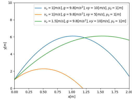
図 2.1: 放物線
