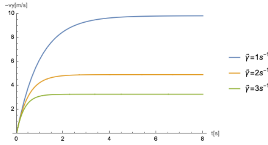
図 4.4: 式 4.18 で与えられる運動をいくつかの \tilde{\gamma} について描いた。 g = 9.8 \text{ m/s}^2 , v_0 = 0 \text{ m/s} とした。
