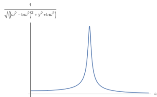
図 4.7: 強制振動における特解の振幅を外力の振動数 \omega の関数として描いた。
