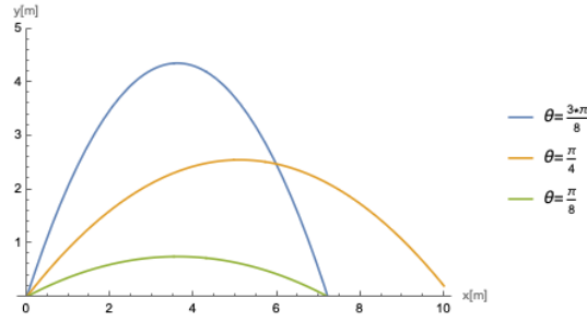
図 4.2: 式 4.13 で与えられる放物線をいくつかの角度 \theta について描いた。 g = 9.8m/s^2, v_0 = 10m/s とした。
