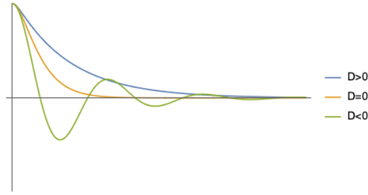
図 4.6: 減衰振動における過減衰、臨界減衰、減衰振動の例を描いた。 x(0) = 1, \dot{x}(0) = 0 とした。
