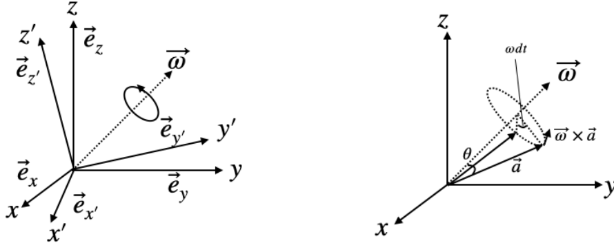
図 8.3: 一般の回転座標系
