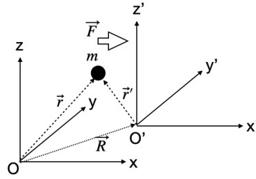
図 8.1: 慣性系と運動座標系
