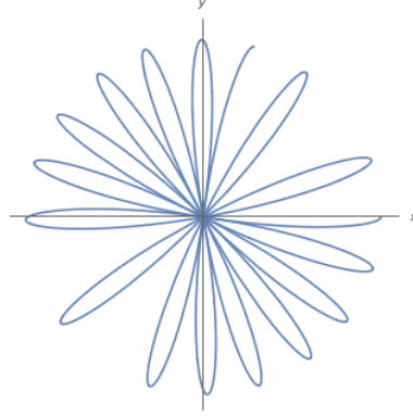
図 8.4: フーコーの振り子が描く軌道の例
