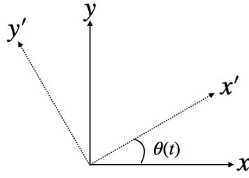
図 8.2: 回転座標系
