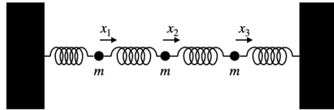
図 9.5: 連成振動のモデル
