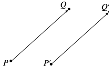
Figure1.2 \vec{PQ} と \vec{P'Q'} は同じ向きで同じ長さの有向線分であるので、同じベクトルとみなされる。
