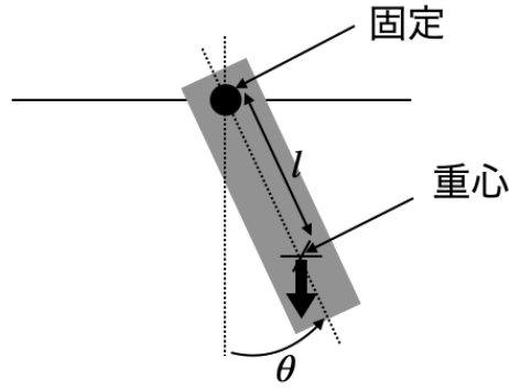
Figure 10.2 物理振り子の模式図
