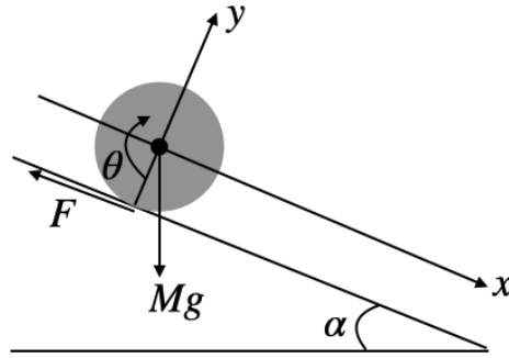
Figure10.3 斜面を転がる円筒の模式図
