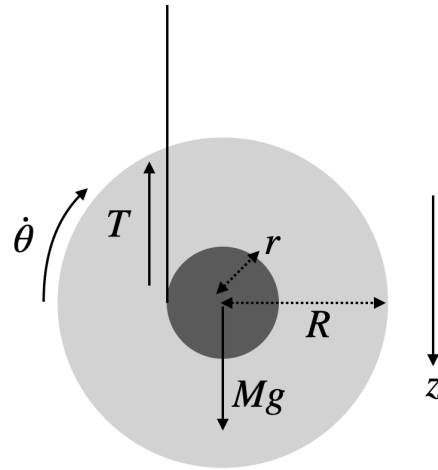
Figure10.4 ヨーヨーの模式図
