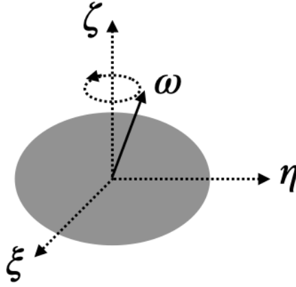
Figure 11.2 地球の歳差運動
