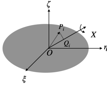
Figure 11.1 任意の回転軸 OX を持つ剛体の回転
