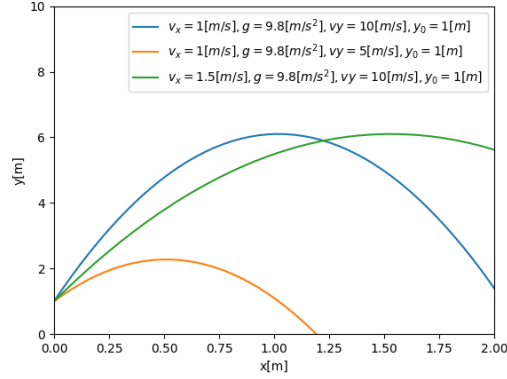
Figure2.1 放物線
