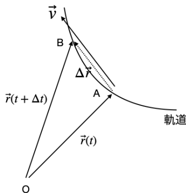
Figure 2.3 質点の速度
