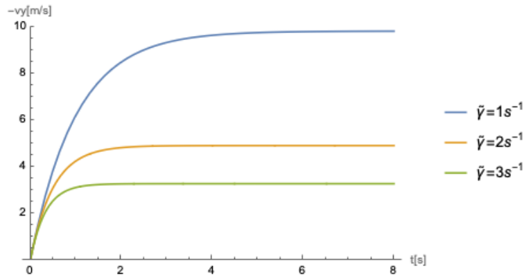
Figure4.4 式 4.18 で与えられる運動をいくつかの \tilde{\gamma} について描いた。 g = 9.8\text{m/s}^2, v_0 = 0\text{m/s} とした。
