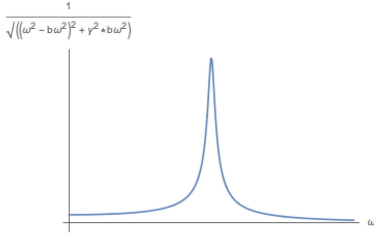
Figure 4.7 強制振動における特解の振幅を外力の振動数 \omega の関数として描いた。
