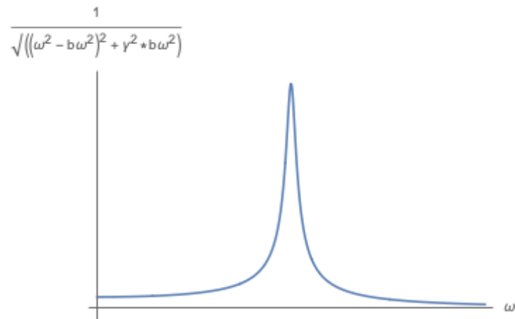
Figure4.7 強制振動における特解の振幅を外力の振動数 \omega の関数として描いた。
