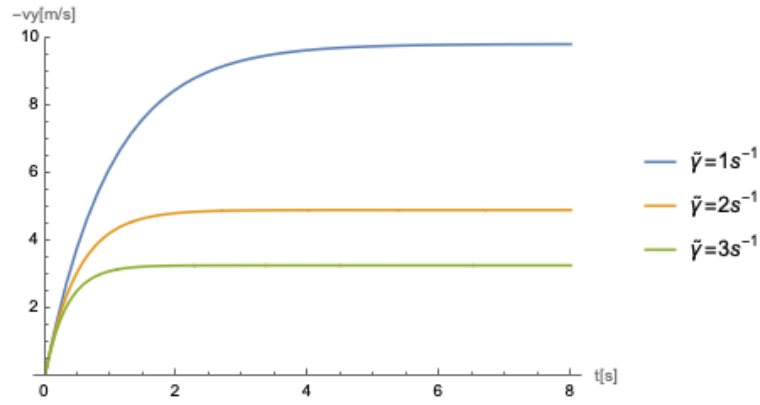
Figure4.4 式 4.18 で与えられる運動をいくつかの \tilde{\gamma} について描いた。 g = 9.8\text{m/s}^2, v_0 = 0\text{m/s} とした。
