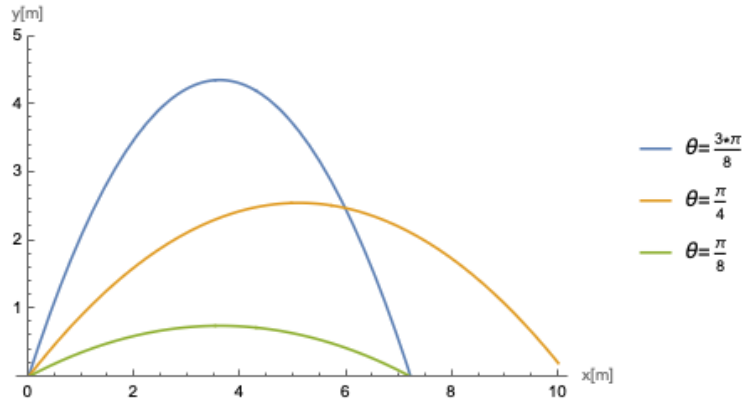
Figure4.2 式 4.13 で与えられる放物線をいくつかの角度 \theta について描いた。 g = 9.8m/s^2 , v_0 = 10m/s とした。
