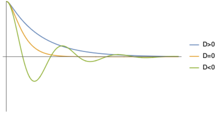
Figure 4.6 減衰振動における過減衰、臨界減衰、減衰振動の例を描いた。 x(0) = 1, \dot{x}(0) = 0 とした。
