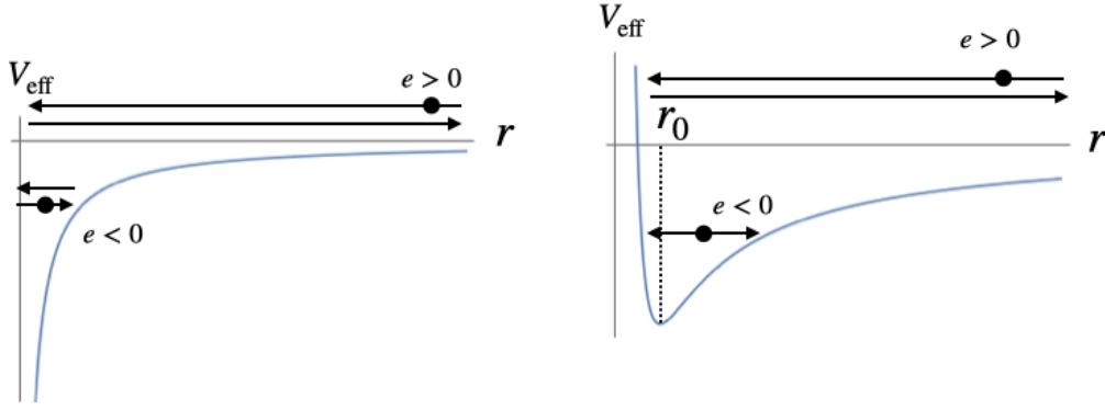
Figure 7.2 有効ポテンシャルの形状。左は l = 0 の場合、右は l \neq 0 の場合を示す。
