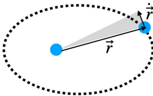
Figure 7.1 面積速度の図示
