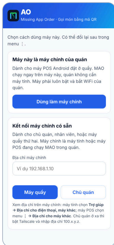
Hình 2. Mở app MAO lần đầu — Chọn làm máy chính hoặc kết nối máy chính có sẵn
