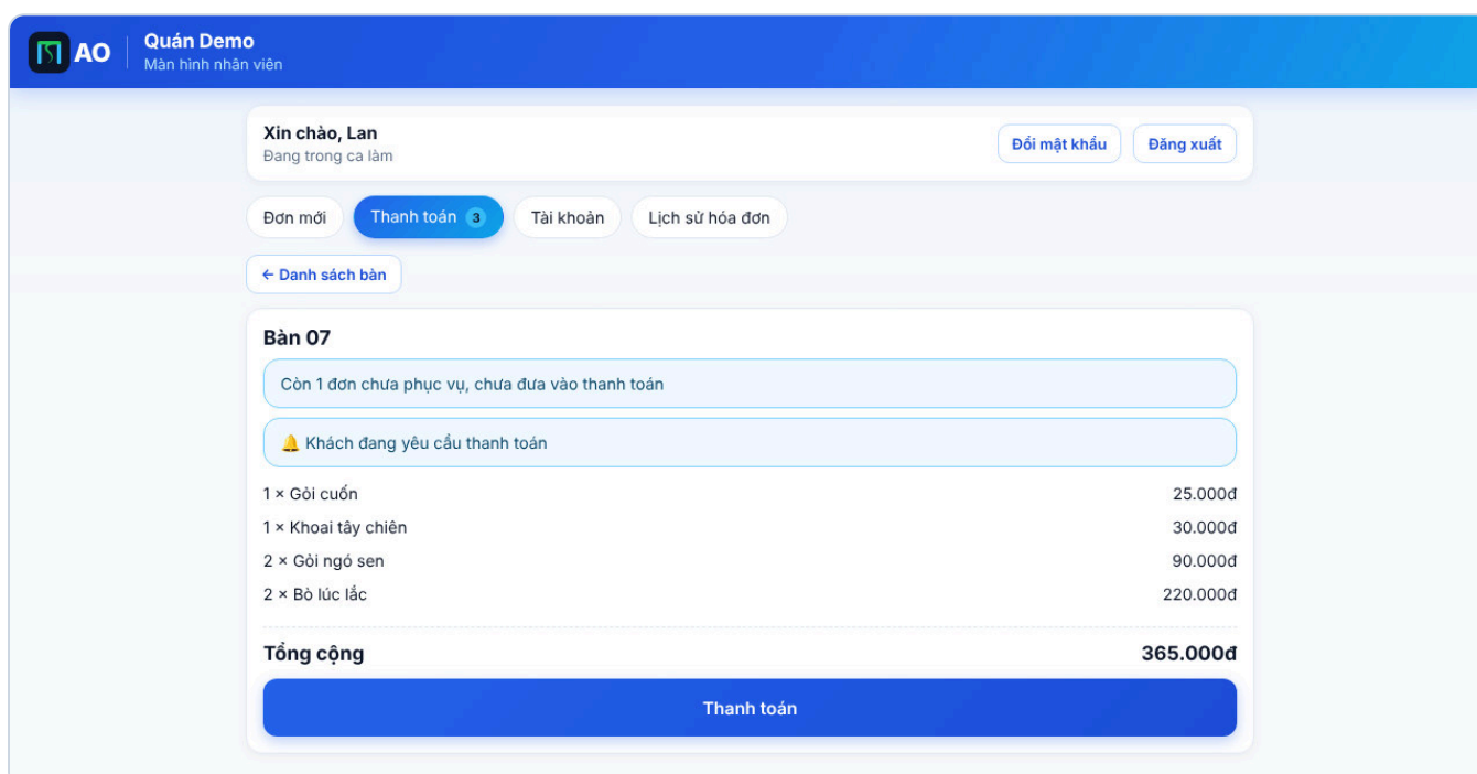
Hình 18. Chi tiết bàn — Chỉ món đã phục vụ mới được tính tiền
