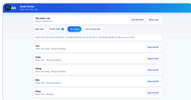
Hình 22. Tài khoản nhân viên — Cấp mã vào ca cho nhân viên khác
