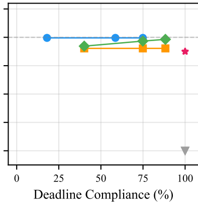
Mistral-7B
