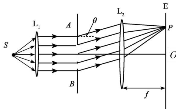
图 1 夫琅禾费单缝衍射缝衍射原理图
