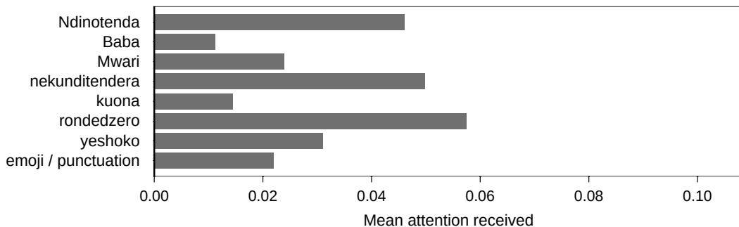
(b) AfroXLMR
