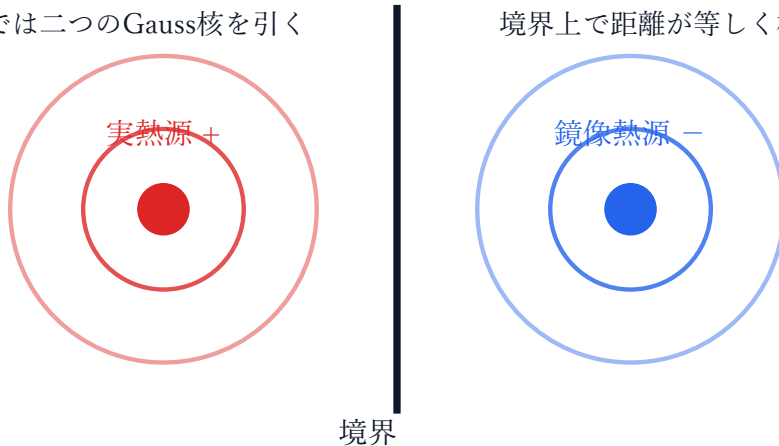
図 11: Dirichlet 境界の鏡像法。負の鏡像熱源が境界上で Gauss 核を相殺する。
