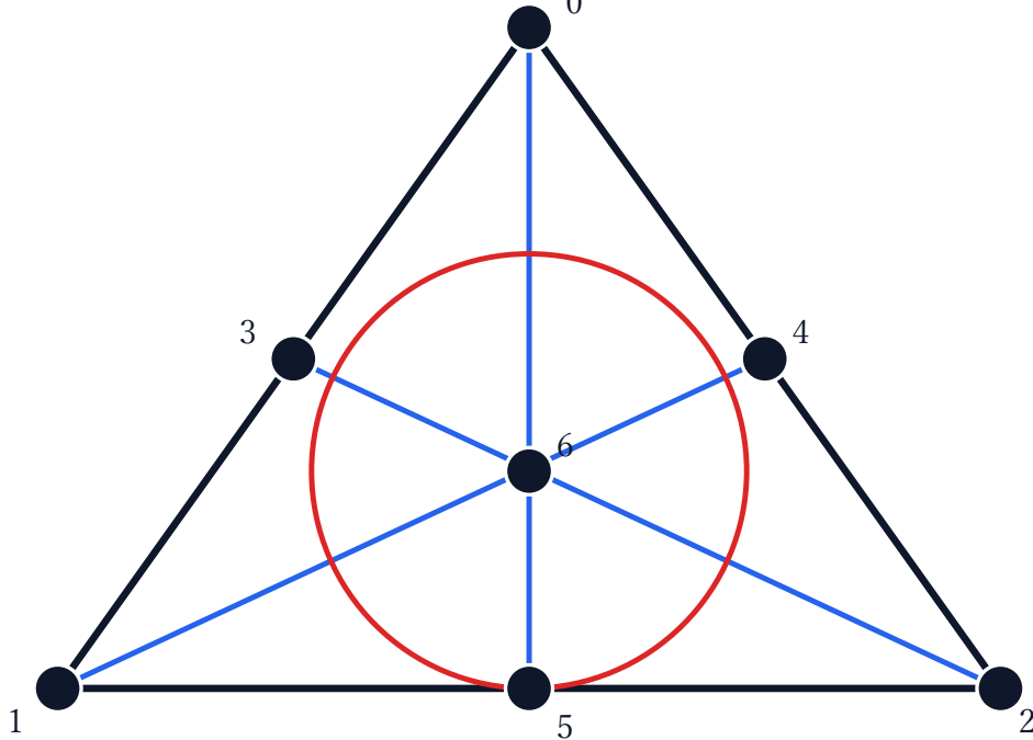
図 20: Fano 平面の 7 点と 7 直線。円も有限幾何では一つの直線を表す。
