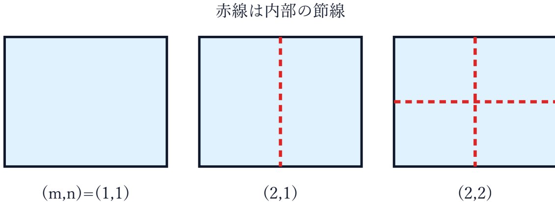
図 5: 長方形モードの節線。符号の異なる領域は逆位相で動く。
