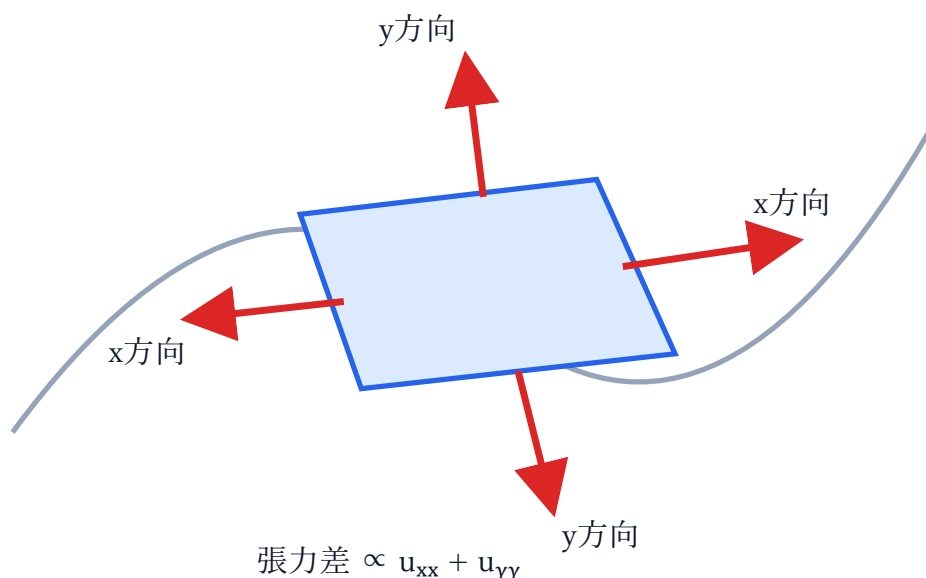
図 3: 膜の微小片。四辺の張力の鉛直成分を足すと Laplacian が現れる。
