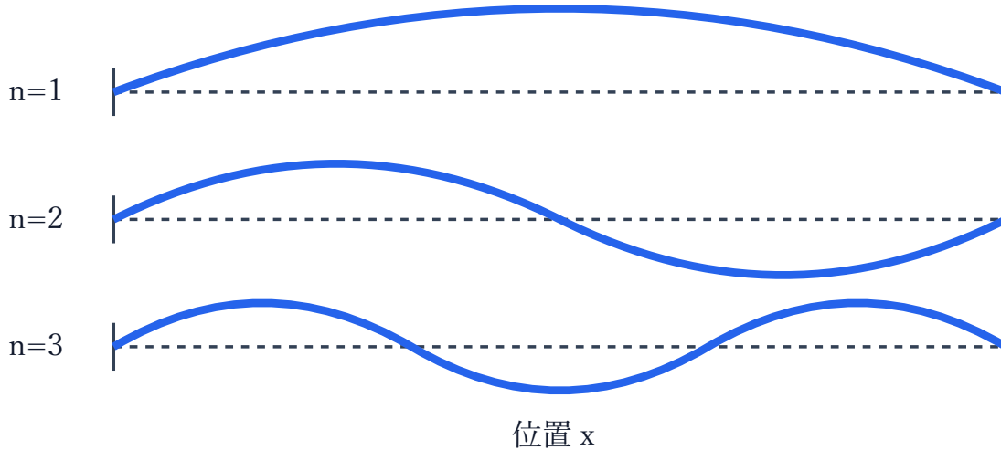
図 2: 固定端弦の最初の三つのモード。
