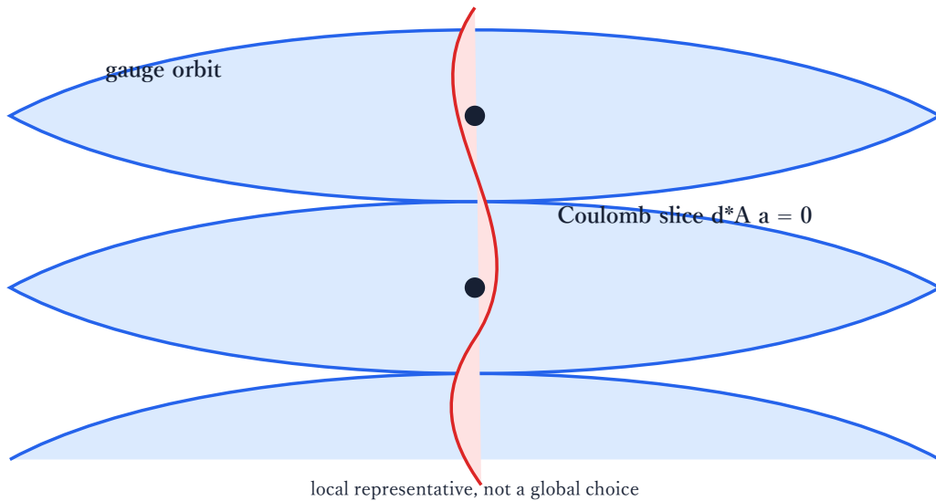
図 3: 接続空間を走る gauge orbit と、それに横断する局所 Coulomb slice。
