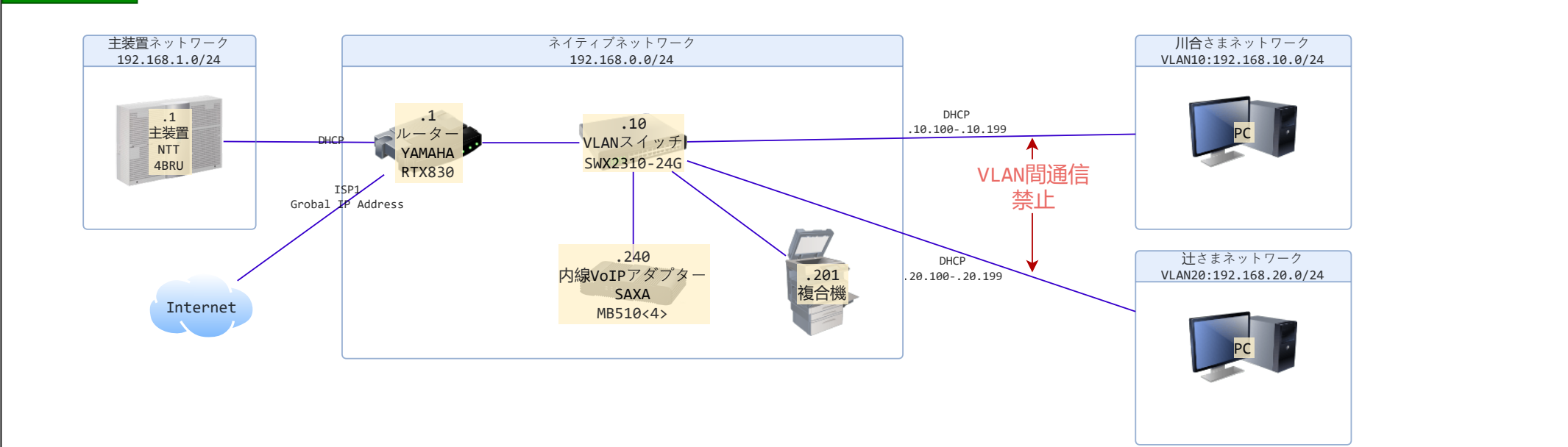
論理構成図
