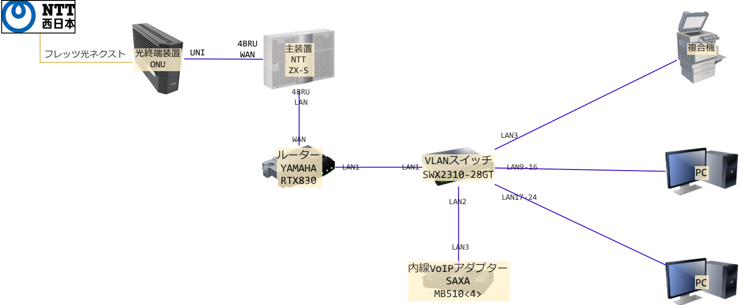
物理配線図
