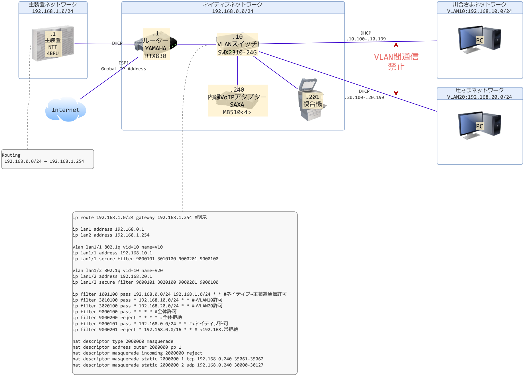
論理構成図
