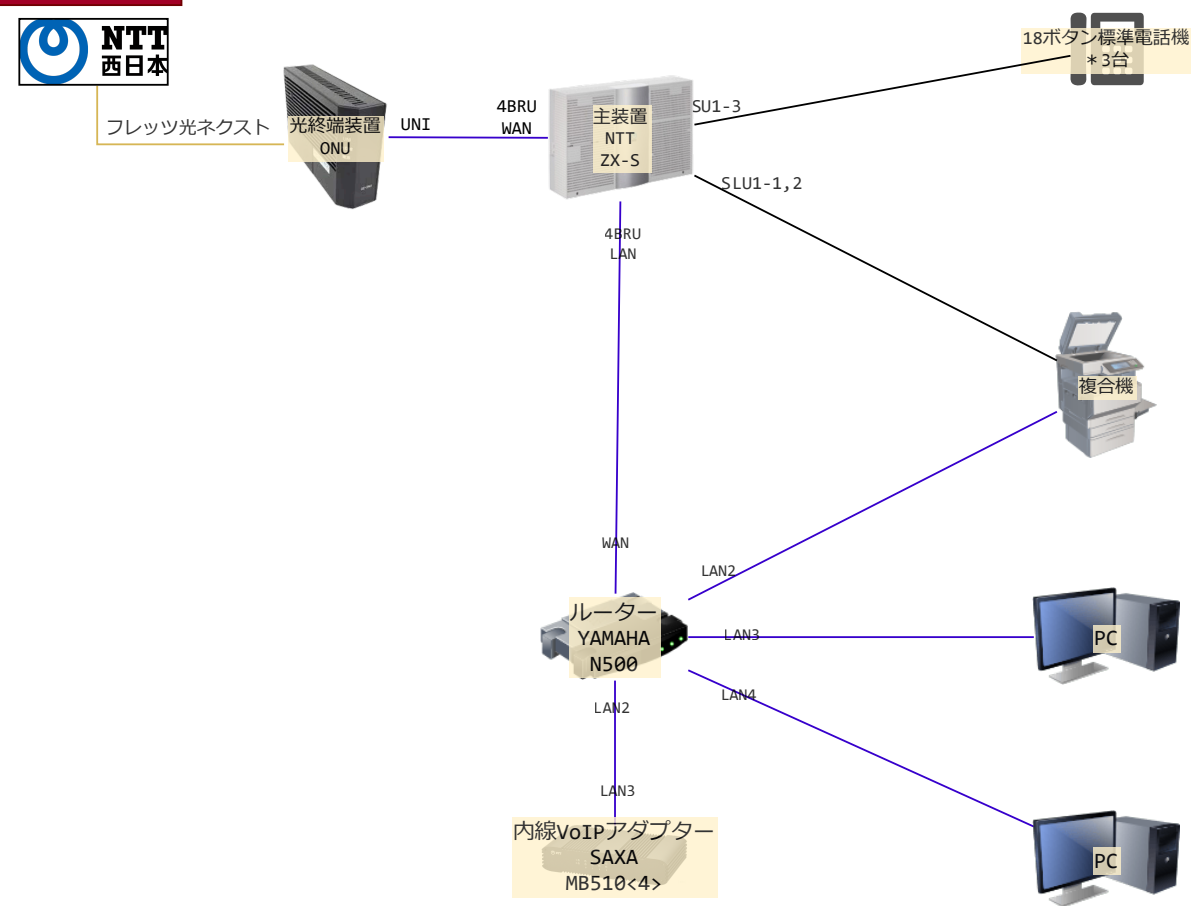
物理配線図
