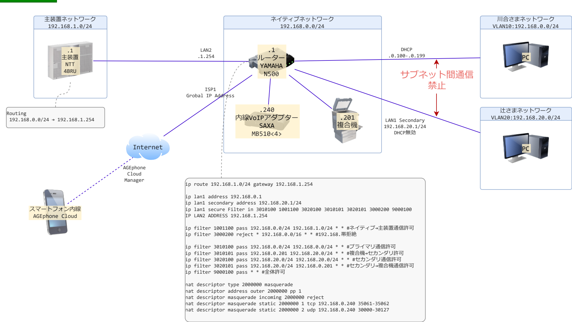
論理構成図
