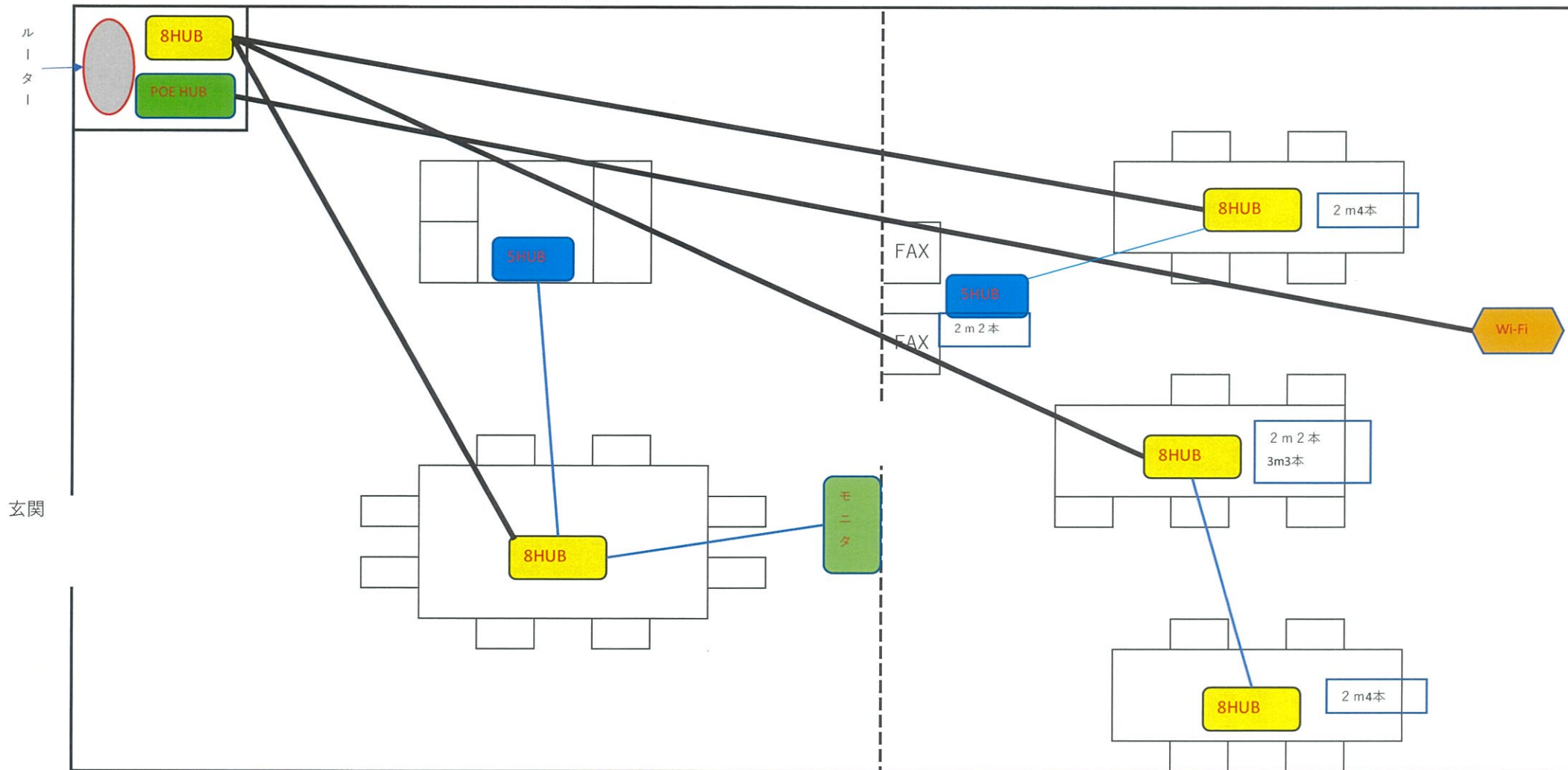
本社 HUBおよびLANケーブル 配置・配線図
