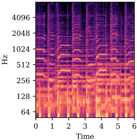
Mixture Y
