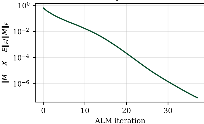
RPCA convergence (38 iters)
