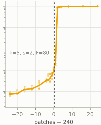
Conv
