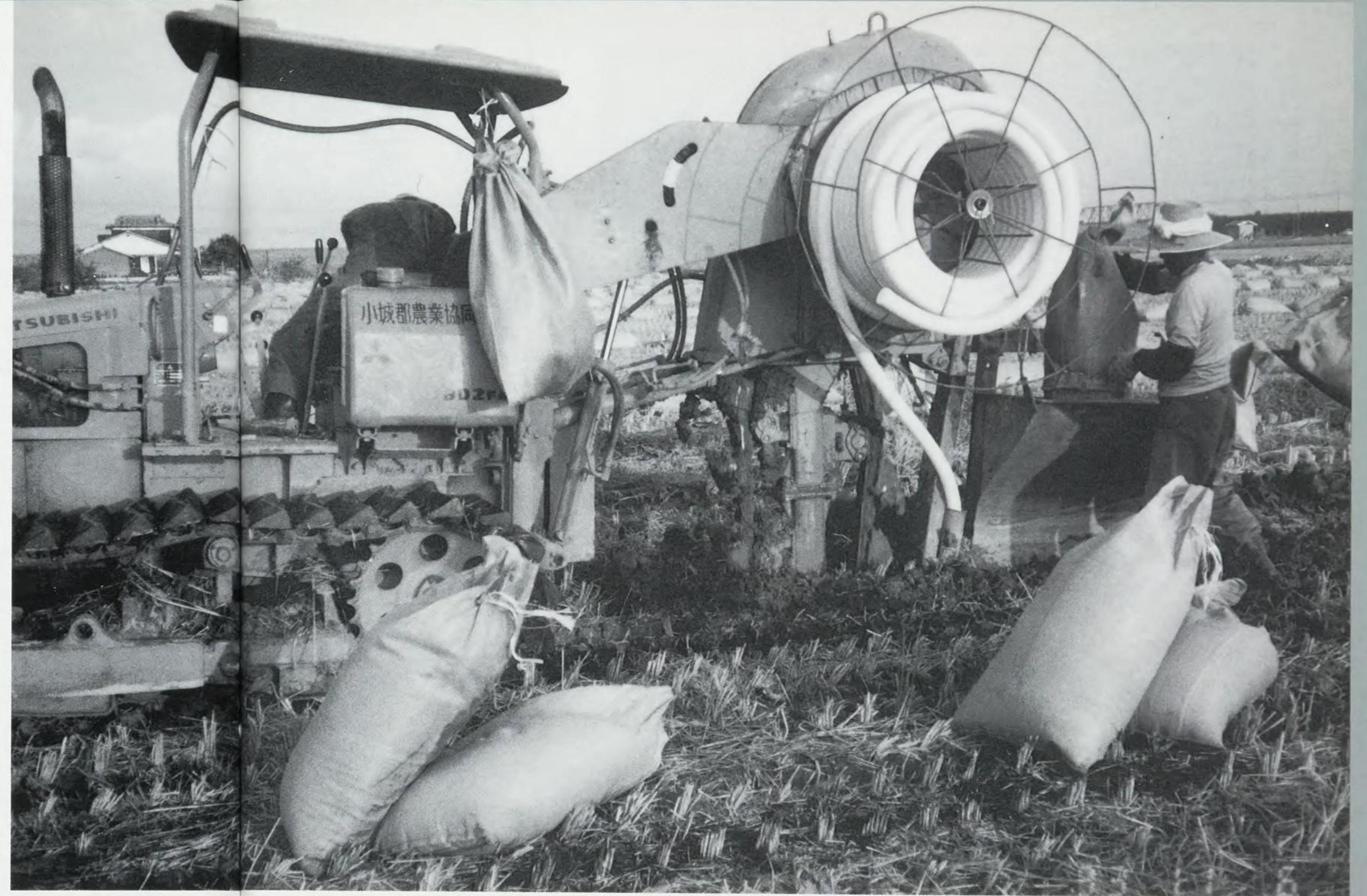
大型トレンチャーによるモミガラ暗渠施工。吸水管とモミガラが掘削と同時に設置できる (佐賀県三日月町 58年11月)
