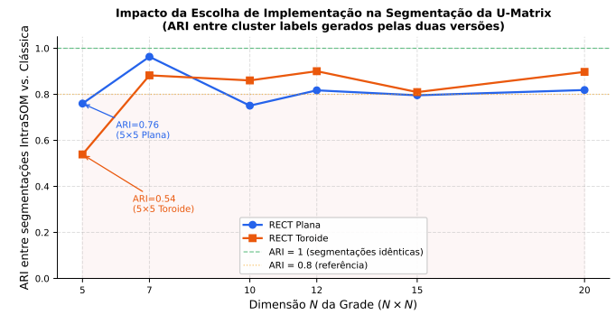
Figura 4. Adjusted Rand Index (ARI) entre segmentações de U_A e U_B ( k = 6 , médias sobre 5 seeds) em função do tamanho da grade.
