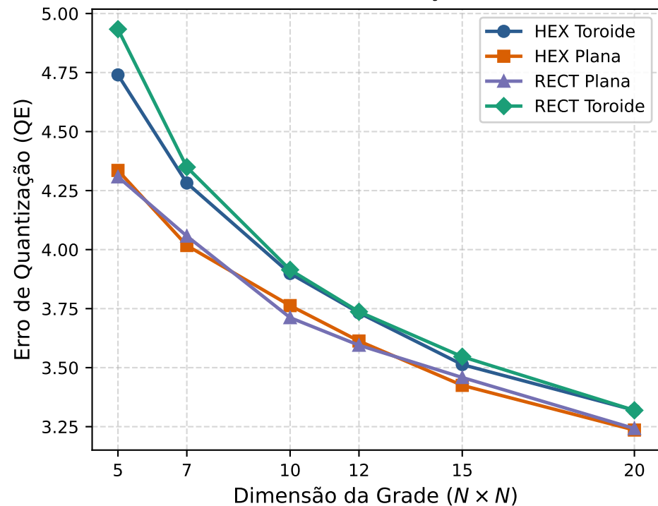
(a) Erro de Quantização ( QE \downarrow )
