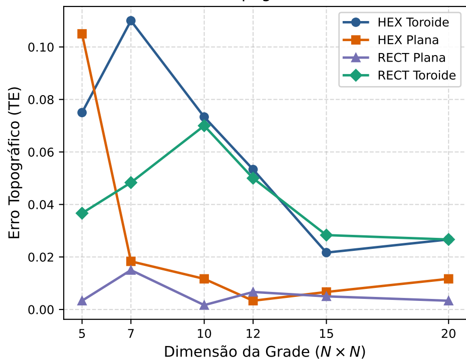
(b) Erro Topográfico ( TE \downarrow )
