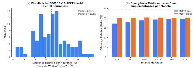
Figura 2. (a) Distribuição da divergência relativa por neurônio para SOM 10 \times 10 RECT toroidal. (b) Diferença relativa média (%) por modelo e topologia (médias sobre 5 seeds).
